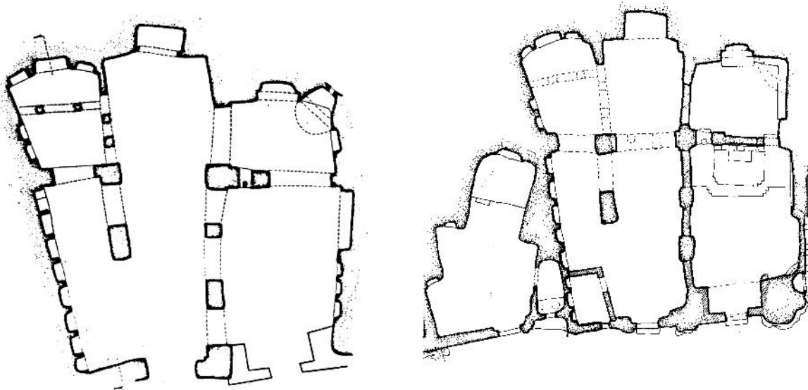
Rilievi della chiesa rupestre di S. Lucia alle Malve prima e dopo i lavori di restauro del 1978.
